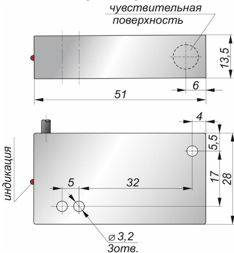
Габаритный чертеж
