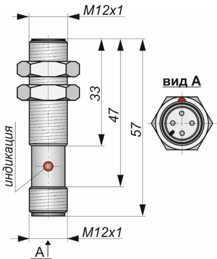
Габаритный чертеж
