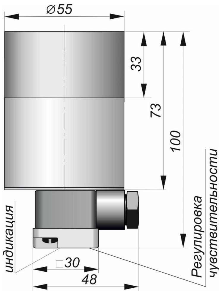
Габаритный чертеж
