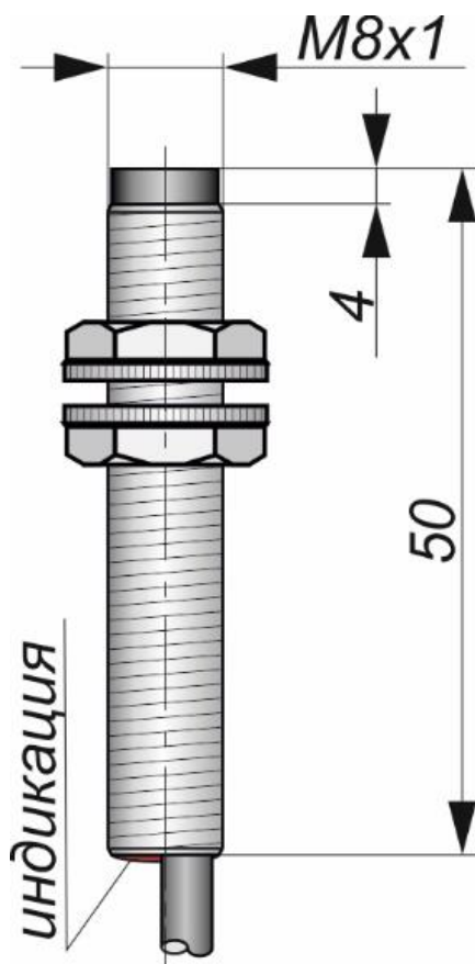
Габаритный чертеж
