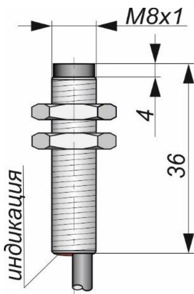
Габаритный чертеж
