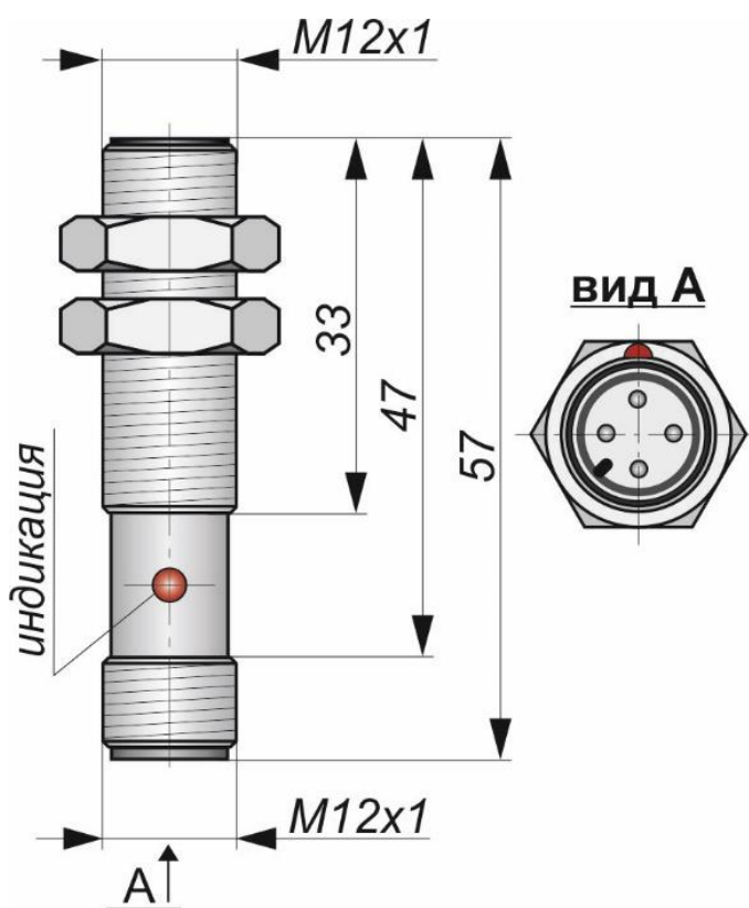
Габаритный чертеж
