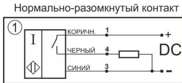
Схема соединения
