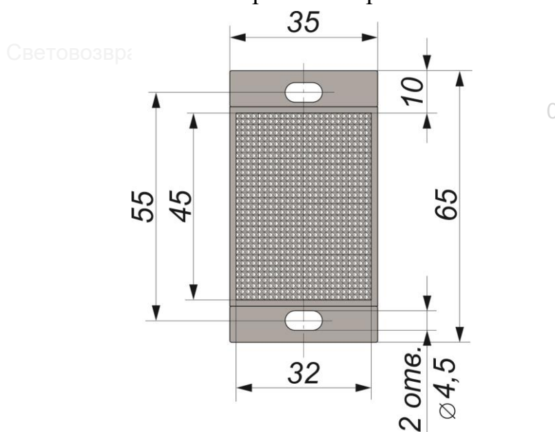
Габаритный чертеж
