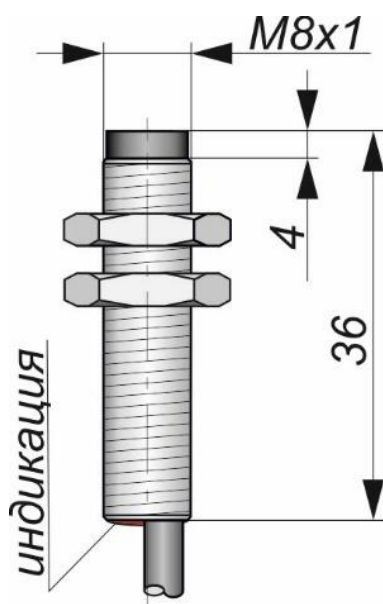
Габаритный чертеж
